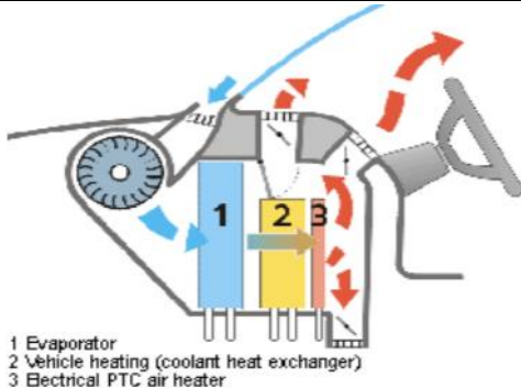
그림 10. PTC 히터의 내연기관 차량내 위치
