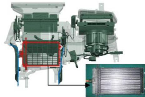
그림 11. PTC 히터의 전기자동차 내 위치
